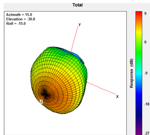
2170MHz
