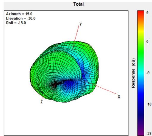
960MHz
