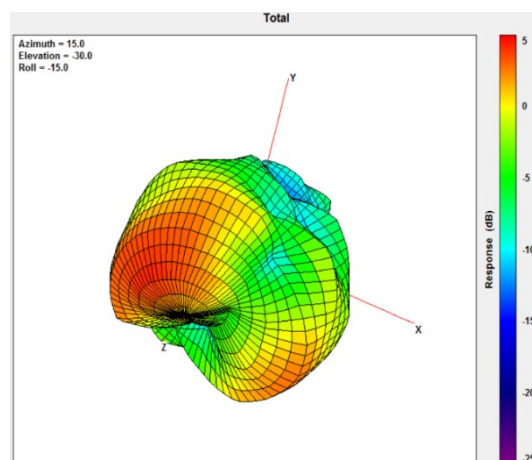
3500MHz
