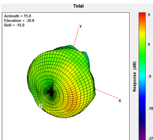
2690MHz
