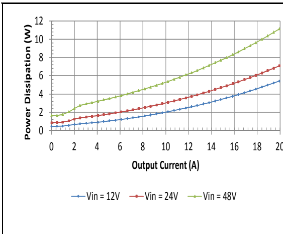
Vo = 3.3V
