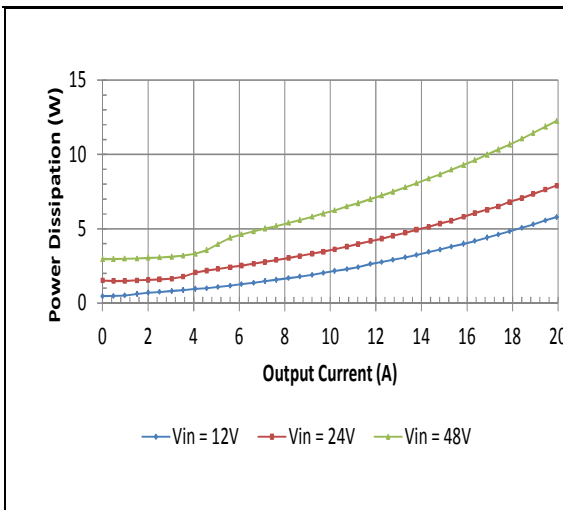
Vo = 9V
