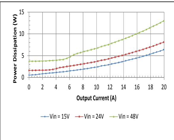
Vo=12V
