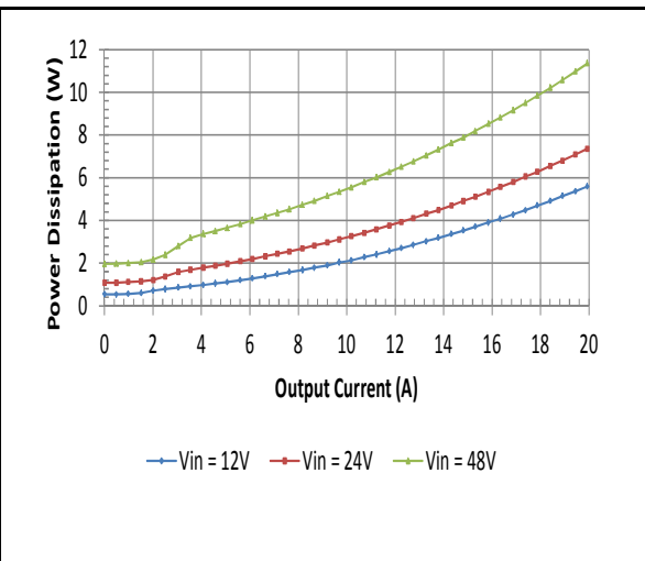
Vo = 5V
