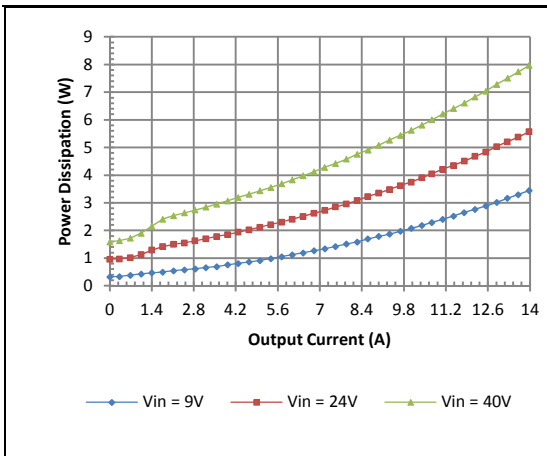
V_o = 5V
