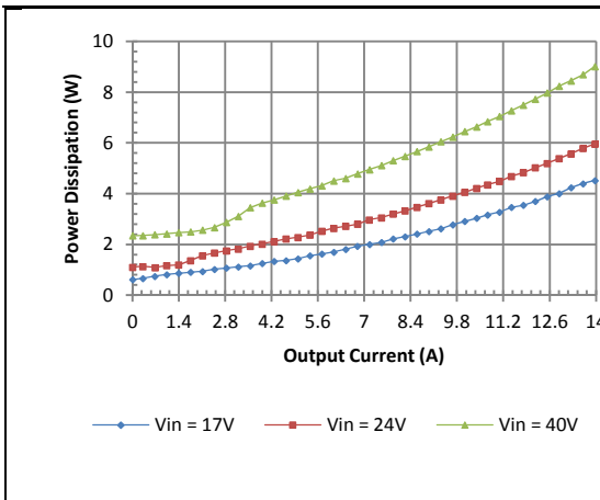
V_o = 15V
