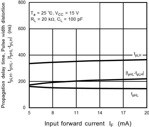
Fig. 13.2.13 t pLH , t pHL , |t pHL - t pLH | - I F
